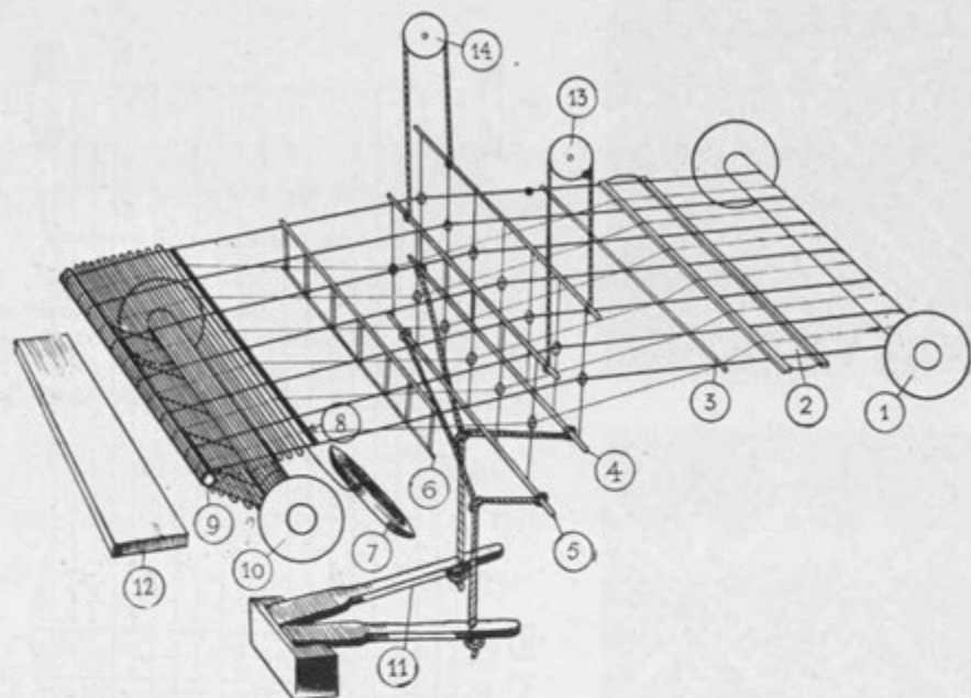
Sl. 11. Shema belokranjskih krosen: 1. gornje vratilo, 2. palici »sestrici«, 3. palica »sklopnjača«, 4. in 5. ničalnice, 6. bilo, v njem brdo, 7. čunek, 8. palica »razpenjalka«, 9. sprednje vratilo, 10. dolnje vratilo, 11. podnožniki, 12. klop, 13. škripci
