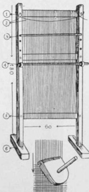
Sl. 13. Gorjanska tara: 1. gornje vratilo, 2. vrvica, 3. palica pomičnica, 4. palica nanitnica, 5. dolnje vratilo, 6. noga; pod taro je češalj (risal T. Ljubič)
