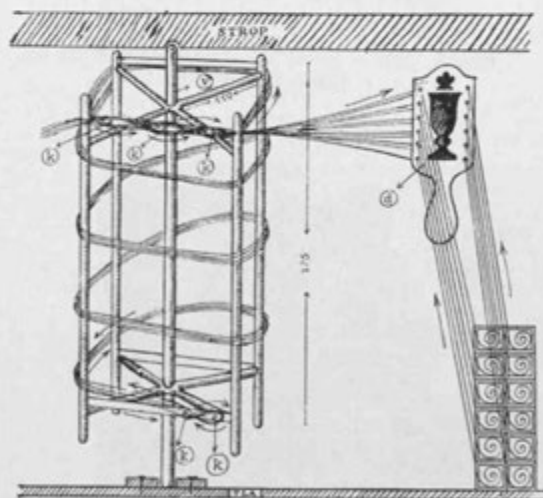
Sl. 12. Vitlen ali snovalo: v = vitlen, k = klinici, d = deščica »snovalka«
