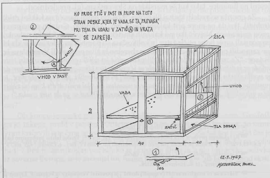
"Vagencja", težnostna komorna past, izpričana v Seniku in v Slepem Vrhovlju. (Risba P. Medvešček, 1957, iz avtorjevega arhiva) ♦ "Vagencja", gravitational box trap, mentioned in Senik and in Slepem Vrhovlje. (Drawing by P. Medvešček, 1957, from the author's archive) ♦ "Vagencja", trappola a peso, documentata a Senik e a Slepem Vrhovlje (Disegno di P. Medvešček, 1957, dall'archivio dell'autore)
