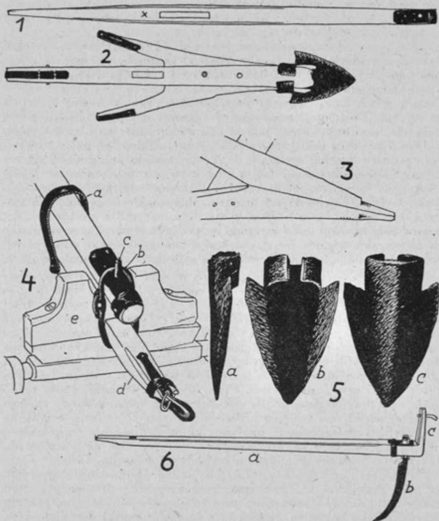
Sl. 2. Deli jezerskega rala: 1. gredal od zgoraj, 2. podsád s peto, lémože in oráunrk od spodaj, 3. sestava lémož in podsada (brez ralnika), 4. del kolc: a rink, b gre-dánca, c cvèk, d sóra z aklom, 5. oráunrk: a s strani, b od spodaj, c od zgoraj, 6. rézounca: a óje, b rézounca, c ročica
