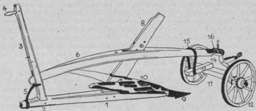
Sl. 1. Ralo »špičmoh« z Jezerskega — sestavni deli: 1. podsád, 2. pěta, 3. ročica, 4. držáu, 5. podpóra, 6. grédal, 7. cvèk, 8. kôzuc, 9. oráunĳk, 10. lémože, 11. poděu, 12. kolesnice, 13. sóra, 14. blazina, 15. rínk, 16. gredánca
