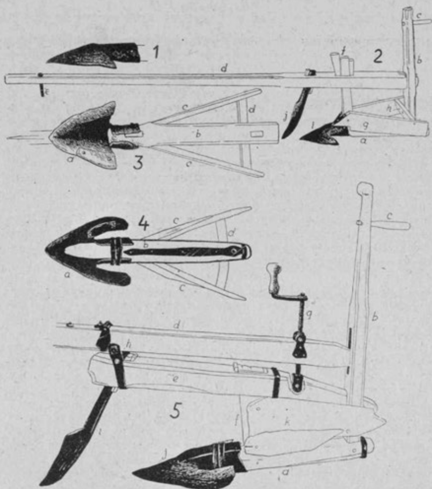
Sl. 4. Ralo na oje iz Srednjega vrha: 1. lémeš S-rala; 2. S-ralo; a puas, b ročica, c držaj, d uóje, e préglej, f stebriček, g uopáte, h vezáva, i lémeš, j črtáu; 3. S-ralo od spodaj; a lémeš, b puas, c uopáte, d vezáva; 4. V-ralo od spodaj; a lémeš, b puas, c uopáte, d vezava; 5. zadnji del V-rala: a puas, b ročica, c držaj, d uóje, e podojnik, f stebriček, g šrauf, h železna os v sponah, i črtáu, j lémeš, k uopáte
